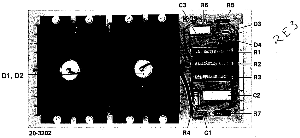
Cathode bias (High voltage regulator power supply) / Kathodenvorspannungseinheit BG 241 241 DS
