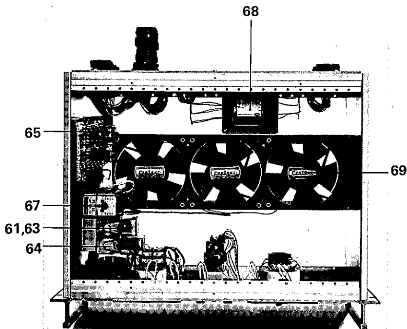
Electron beam power supply / HS-Steuergerät EHV 110 A, U3
